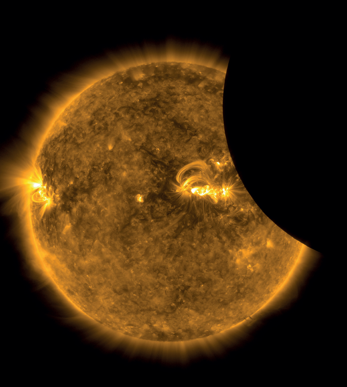
La Luna transitando frente al Sol, tomada por el SDO en luz ultravioleta extrema. NASA/SDO
